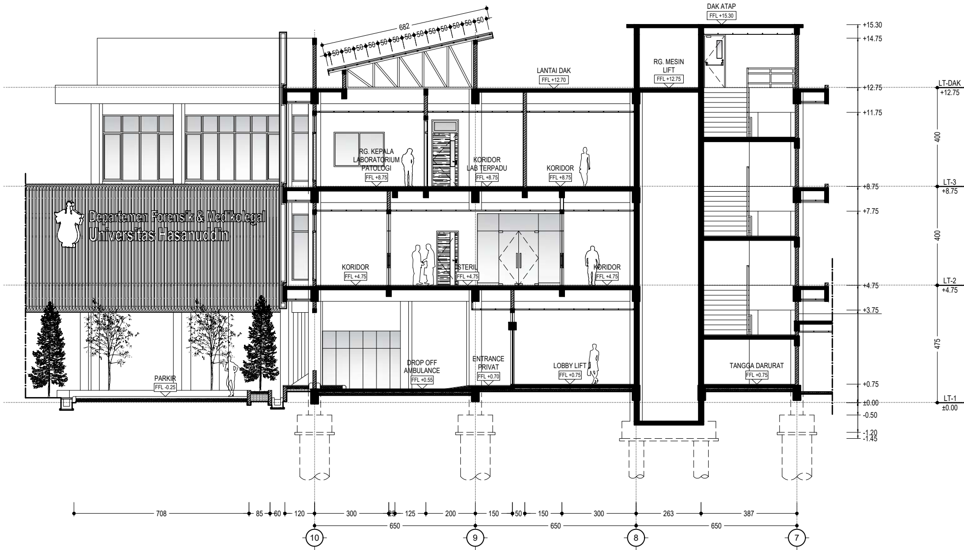
DSG-024 POTONGAN B-B SCALE 1:150
