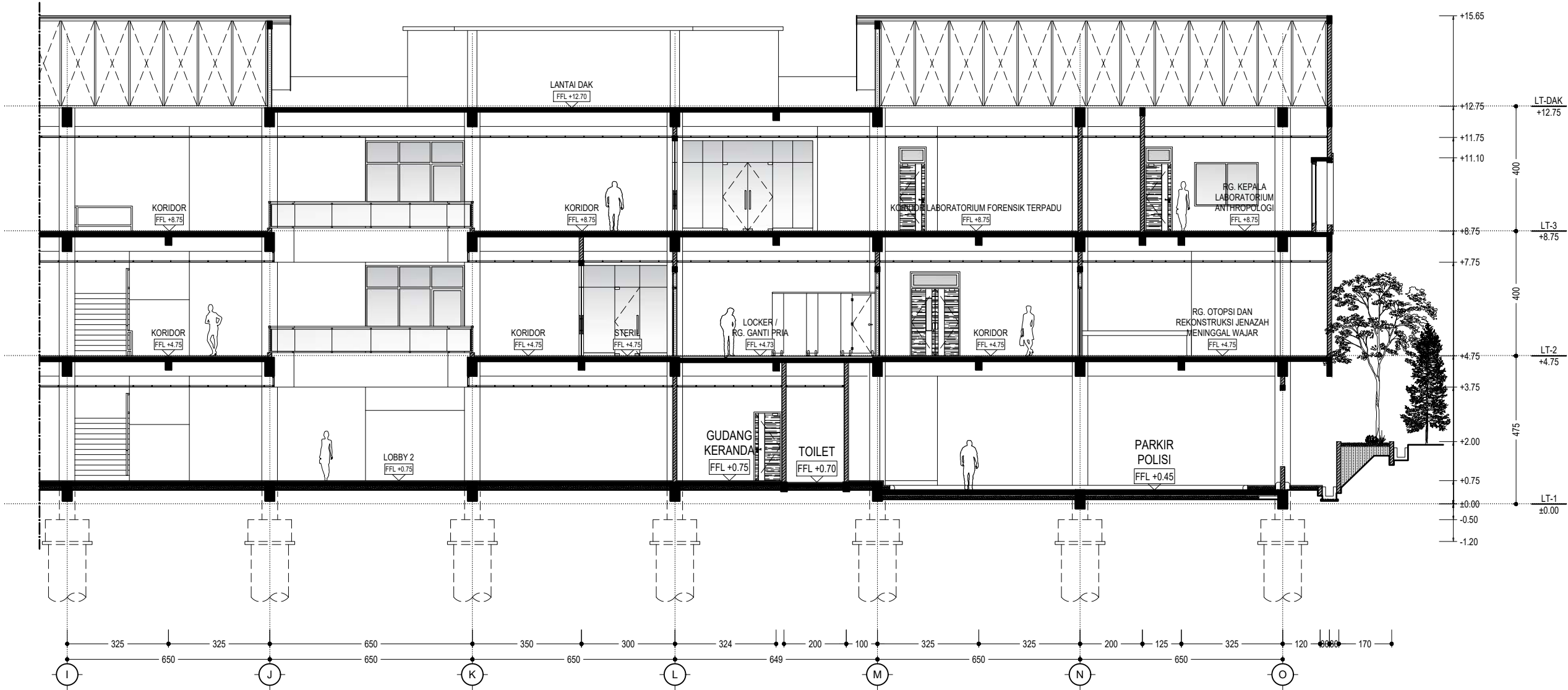
DSG-026 POTONGAN D-D SCALE 1:150
