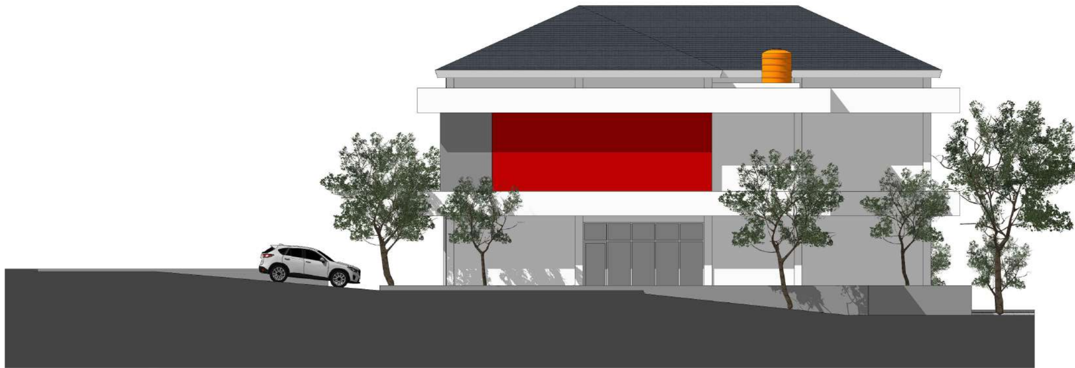
DSG-022 TAMPAK SAMP. KANAN (BANGUINAN ADMINISTRASI) SCALE 1:150
