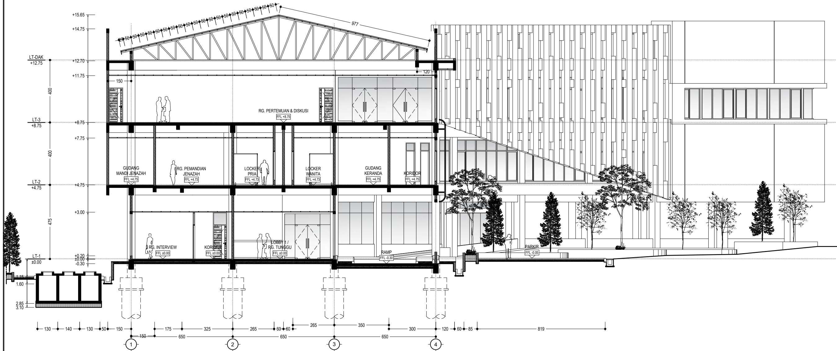
DSG-023 POTONGAN A-A SCALE 1:150
