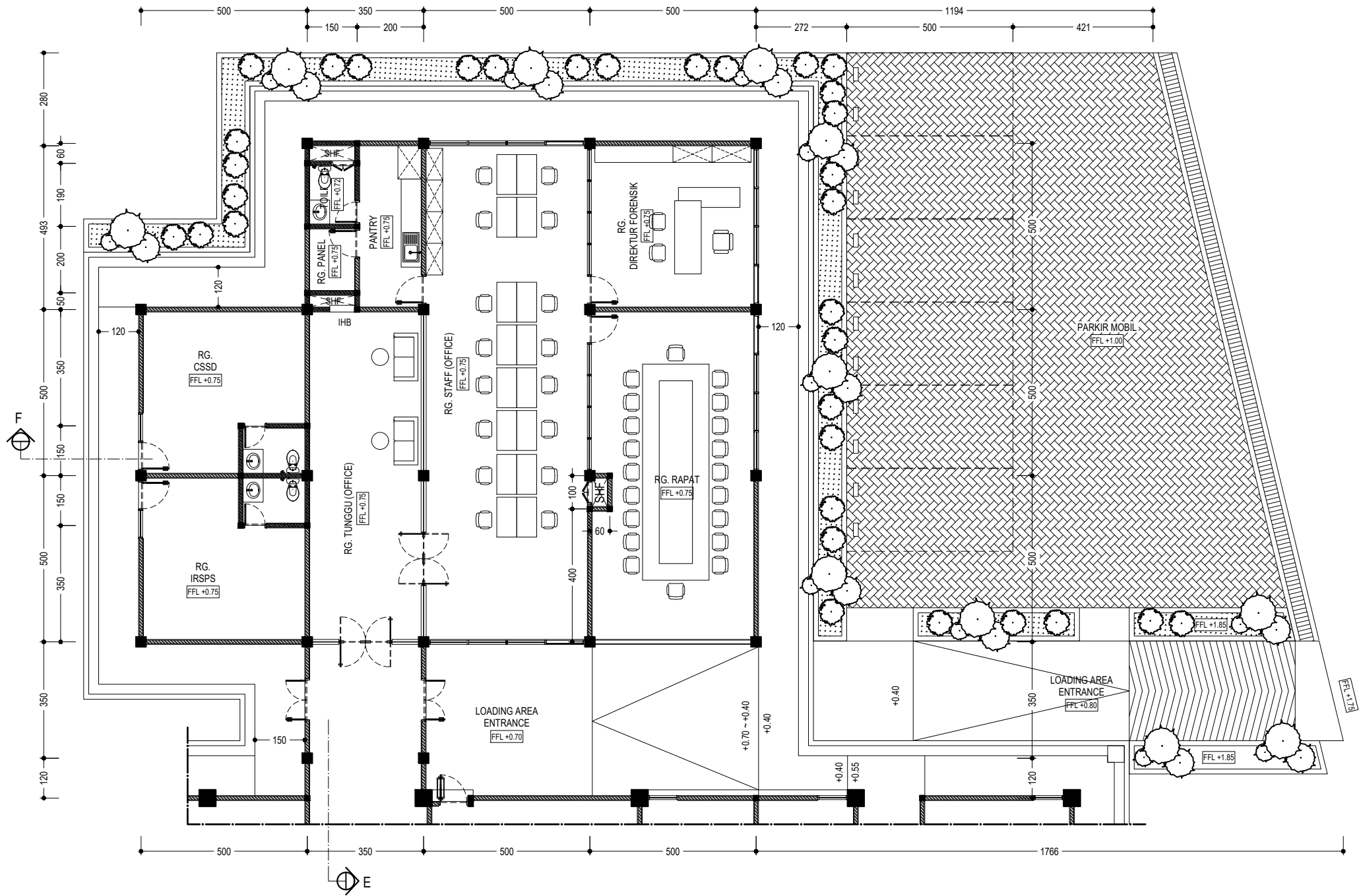
DSG-012 DENAH (BANGUNAN ADMINISTRASI) LT- 1 SCALE 1:150
