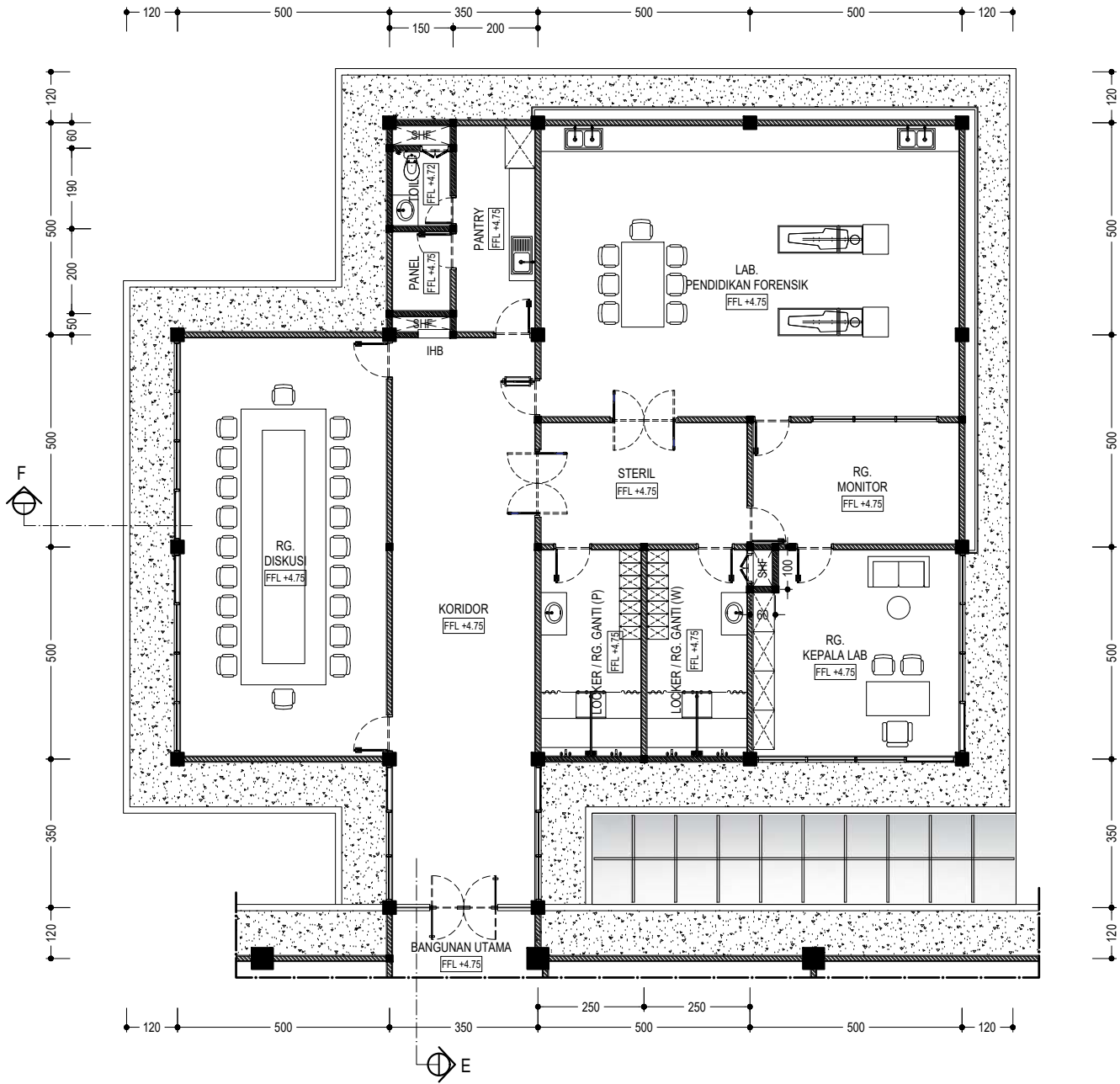
DSG-013 - DENAH (BANGUNAN ADMINISTRASI) LT- 2 SCALE 1:150
